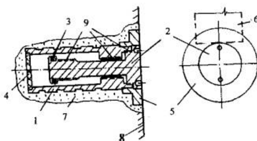
Рис. П.10. Марка закрытого типа конструкции Перепоновой:
