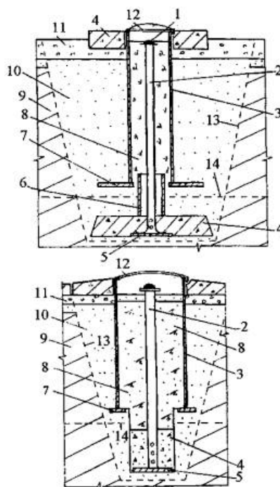
Рис. П.8. Схемы поверхностных постоянных марок:
