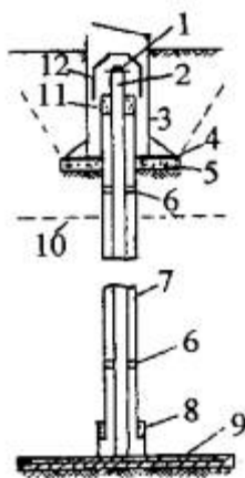
Рис. П.6. Глубинная железобетонная плита-марка:
