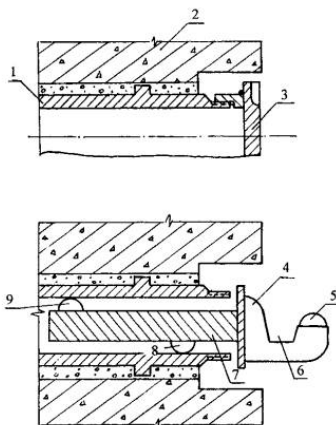
Рис. П.9. Конструкция стенной закладной постоянной марки:
