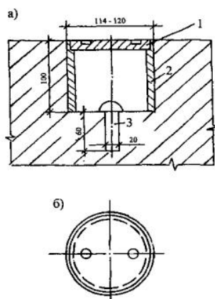
Рис. П.12. Плитная марка (размеры в мм):
