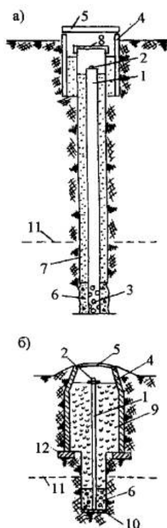
Рис. П.3. Конструкции рабочих реперов для мягких грунтов:
