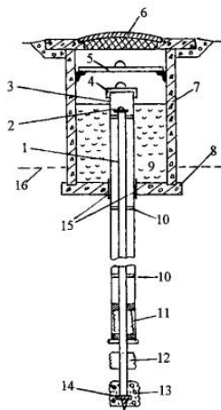
Рис. П.2. Исходный глубинный репер:
