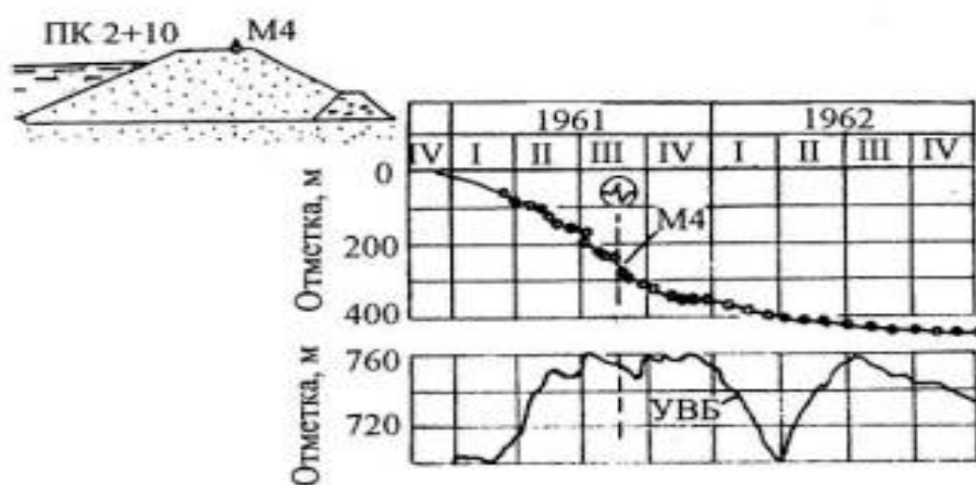
Рис. 6.1. Осадки марки на гребне плотины: ☼ - регистрация землетрясения
