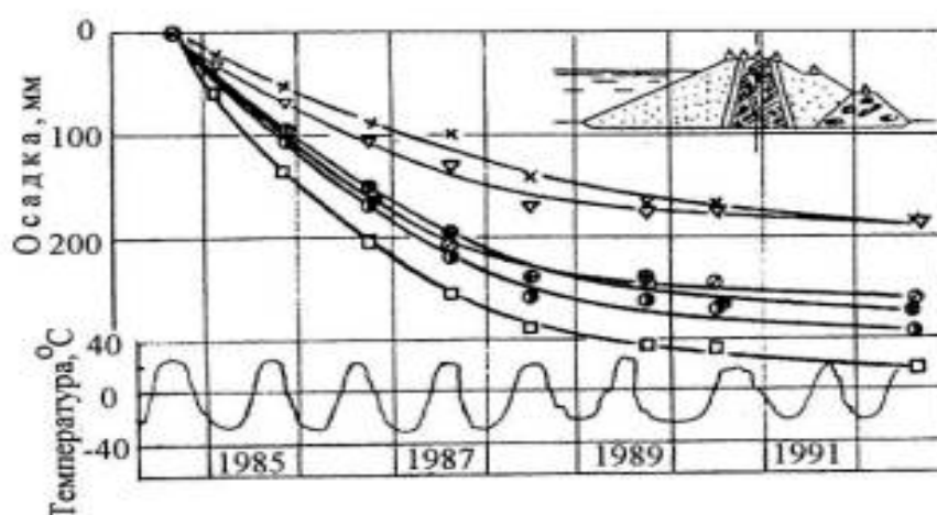
Рис. 6.2. Осадки контрольных марок на гребне грунтовой плотины: □ - M1; Δ - M2; ● - M3; ⊙ - M4; ⊕ - M5; × - M6
