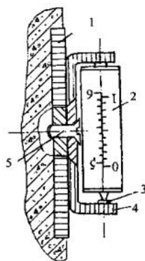
Рис. П.11. Стенная марка конструкции Пискунова:
