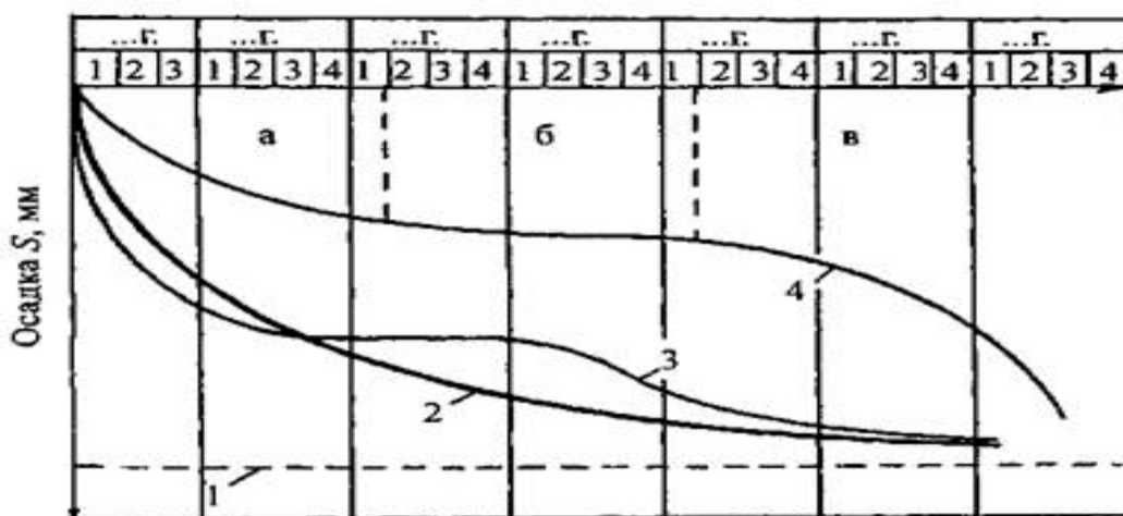
Рис. 7.1. Характерные графики хода осадок во времени:
