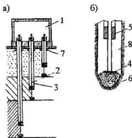
Рис. П.5. Глубинные трубчатые марки:
