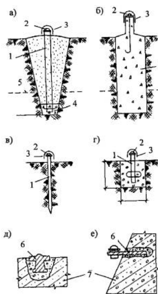
Рис. П.14. Геодезические знаки для установки на обвалоопасных участках и оползнях:
