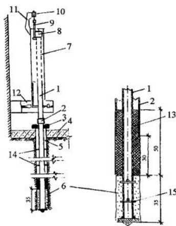
Рис. П.4. Универсальный глубинный репер конструкции Проктора:
