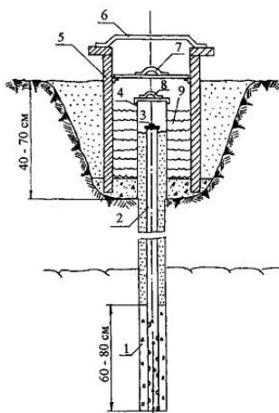
Рис. П.1. Исходный репер трубчатого типа:
