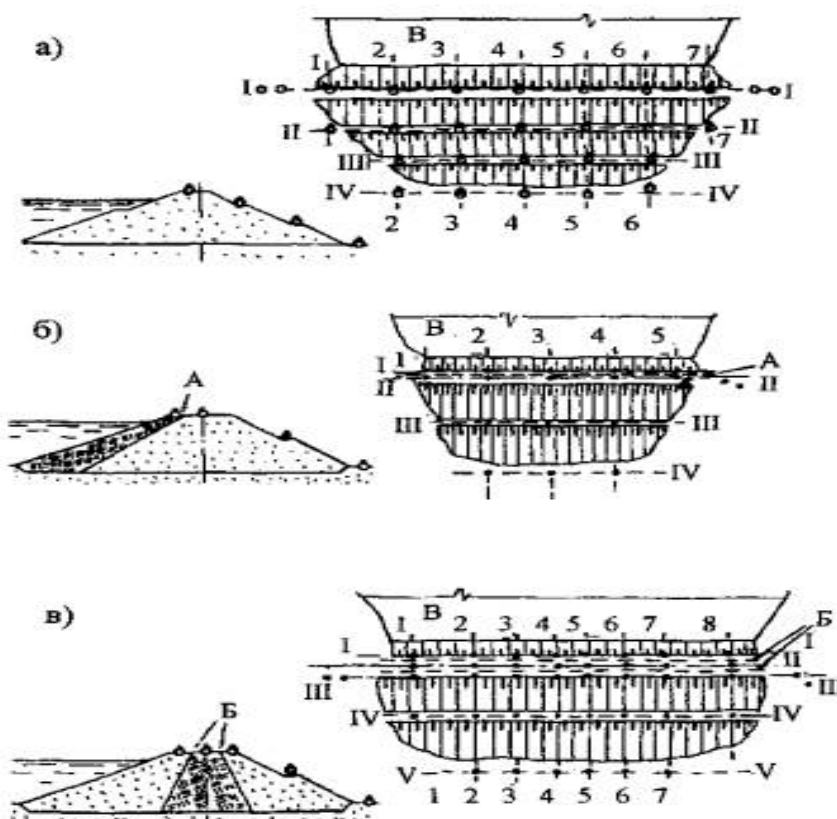
Рис. 4.1. Размещение створов марок в грунтовых плотинах:
