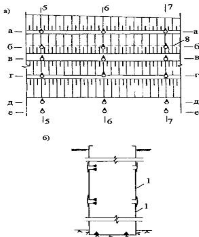
Рис. 4.3. Схема размещения марок в грунтовых плотинах:
