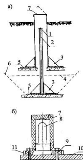
Рис. П.7. Конструкции марок:
