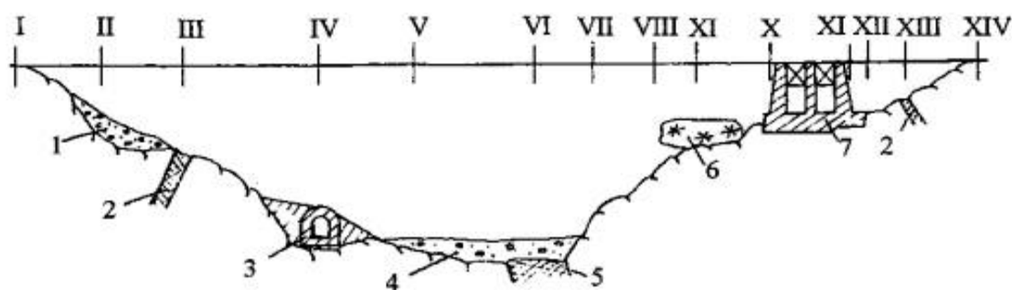
Рис. 4.2. Схема размещения поперечных наблюдательных створов марок:
