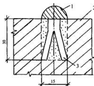
Рис. П.13. Цокольная марка (размеры в мм):
