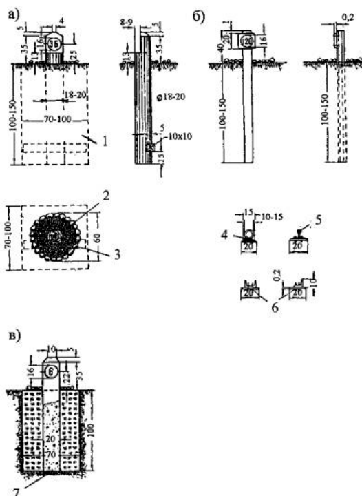
а - деревянный знак; б - металлический знак; в - бетонный знак; 1 - шурф размером 70×100; 2 - галька, щебень; 3 - бордюрный камень; 4 - сварка; 5 - рельс; 6 - заклепки; 7 - подсыпка щебнем или гравием
